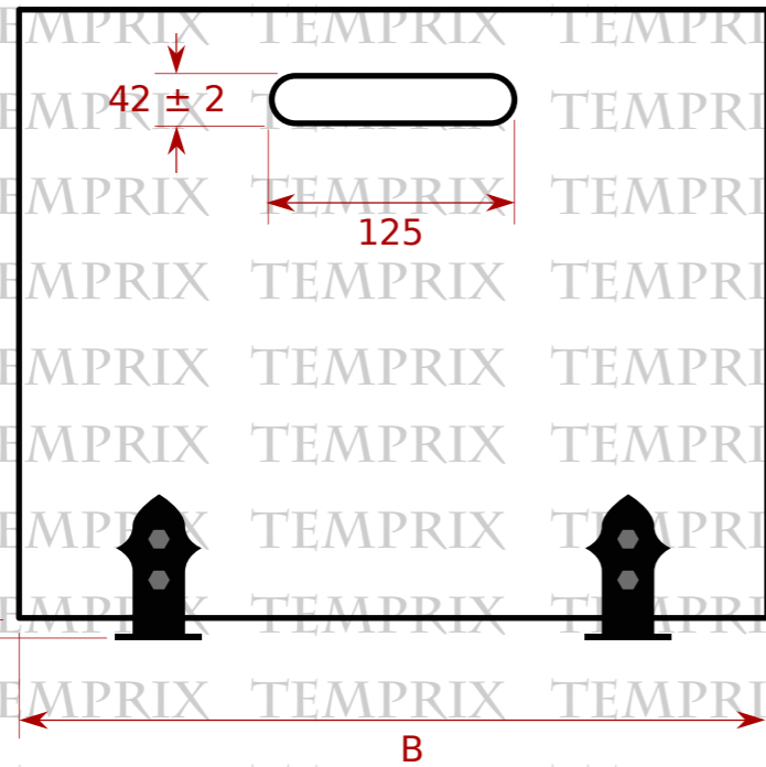
Frontansicht
