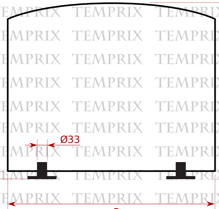
Frontansicht
